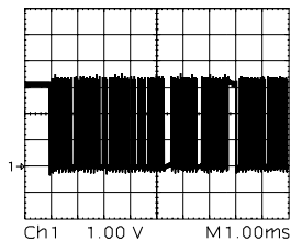
⑤ I2CC (I 2 C-Clock)
